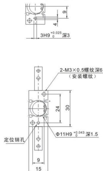
磁性开关安装槽位置
