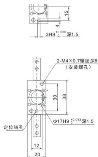
磁性开关安装槽位置
