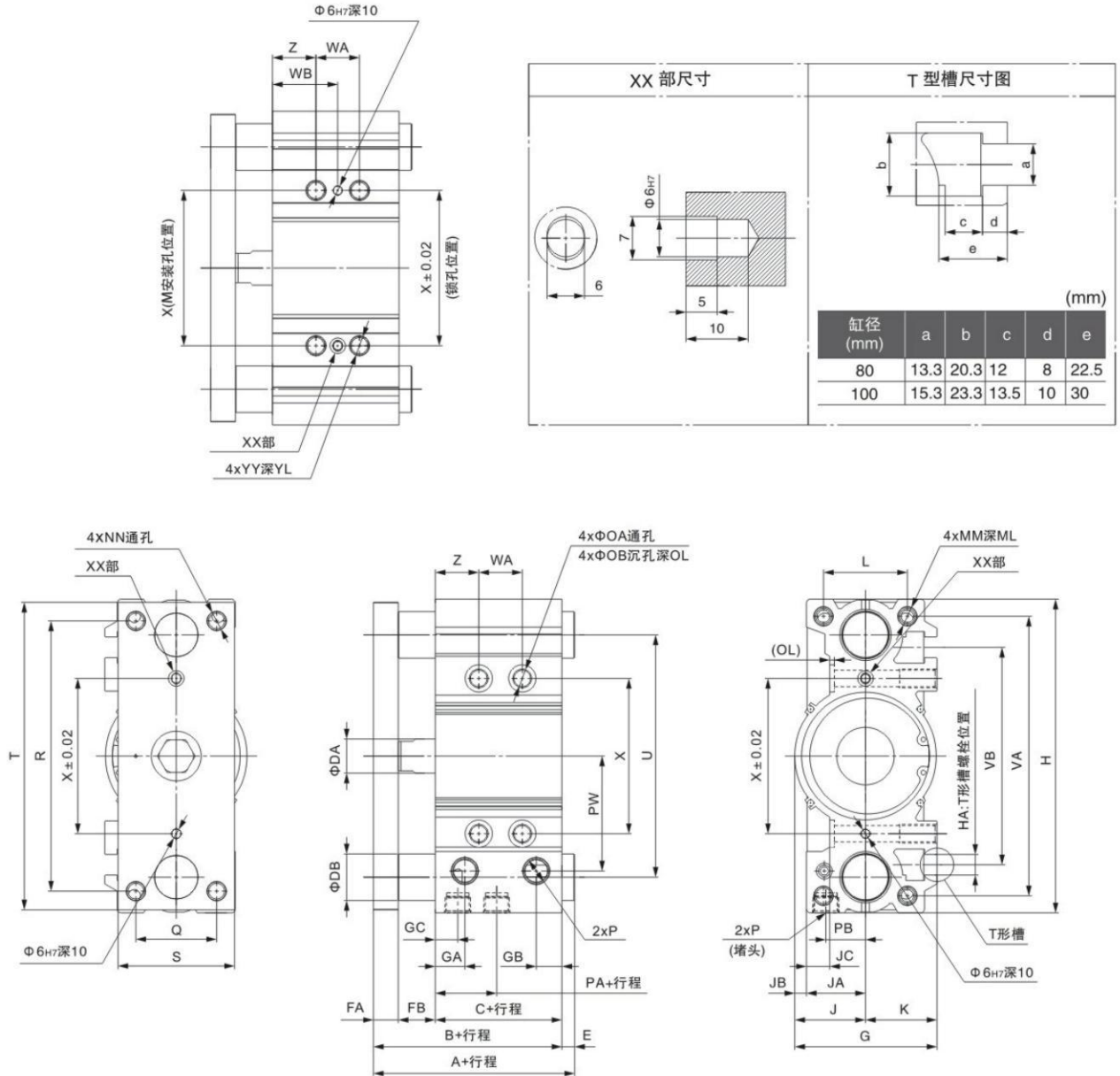
TMGPM, TMGPL 共同尺寸表
