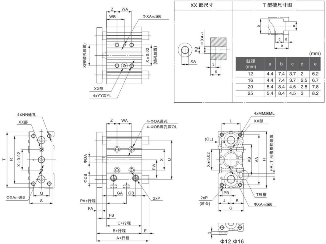
TMGPM, TMGPL共同尺寸表
