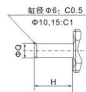
杆端无螺纹情况
